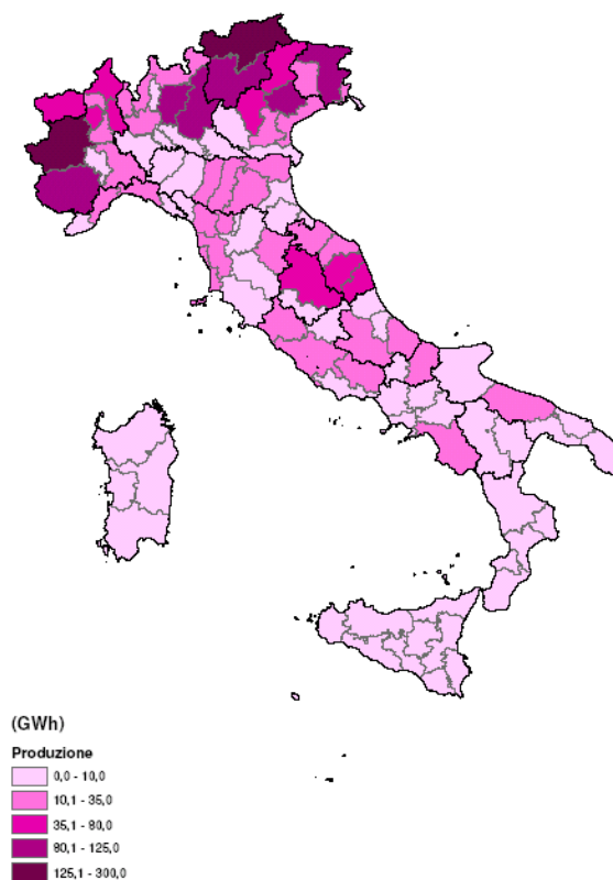
Figura 4.39: Dislocazione degli impianti di MG in termini di energia.
