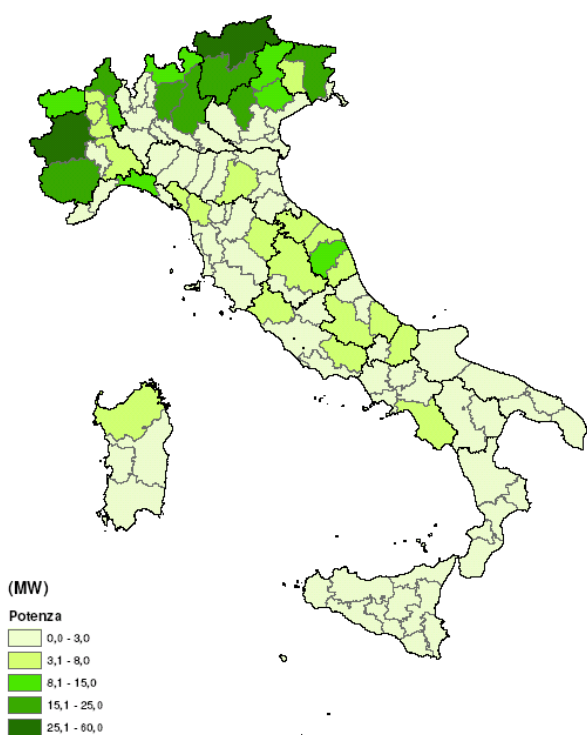
Figura 4.40: Dislocazione degli impianti di MG alimentati da fonti rinnovabili in termini di potenza.
