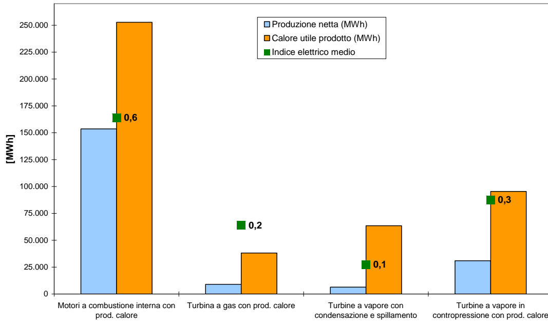
Figura 4.57: Indici elettrici medi per le diverse tecnologie utilizzate per la produzione combinata di energia elettrica e calore nell'ambito della MG.
