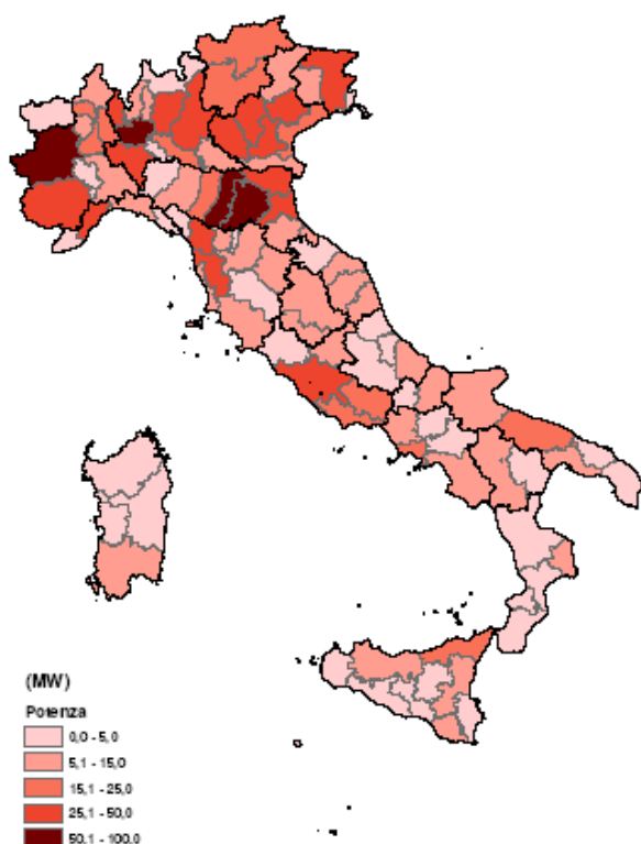
Figura 4.18: Dislocazione degli impianti termoelettrici di GD in termini di potenza.
