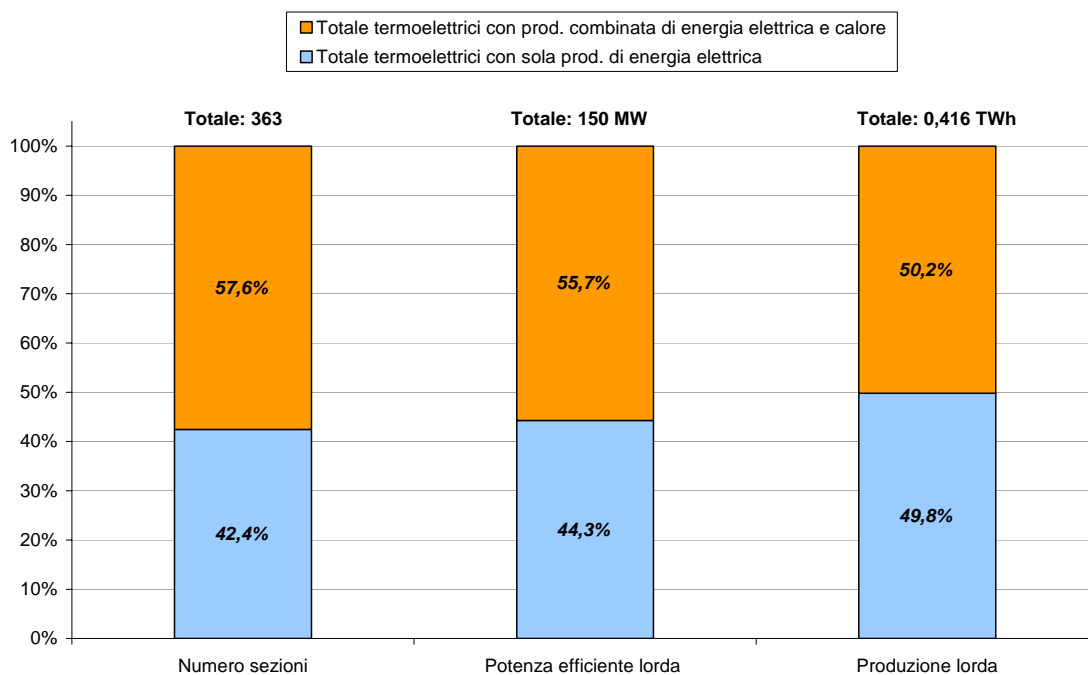
Figura 21: Impianti termoelettrici nell'ambito della MG.
