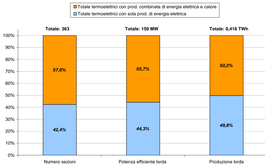
Figura 4.37: Impianti termoelettrici nell'ambito della MG.
