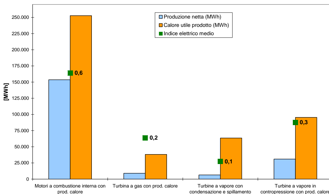
Figura 28: Indici elettrici medi per le diverse tecnologie utilizzate per la produzione combinata di energia elettrica e calore nell'ambito della MG.
