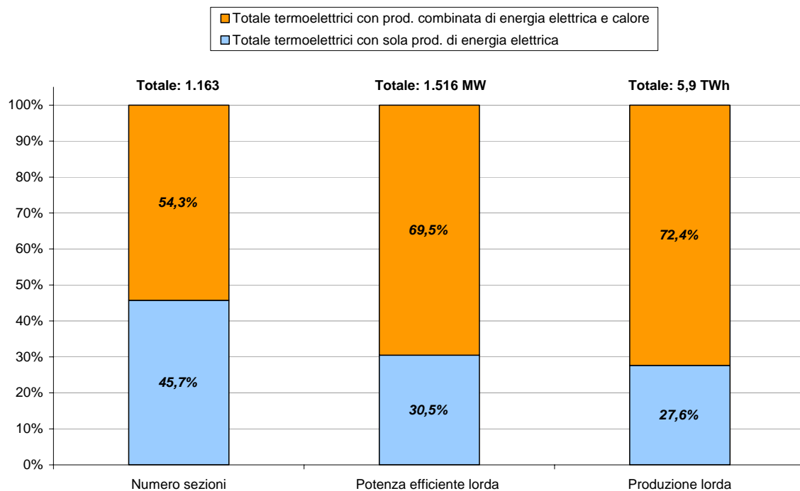
Figura 4.5: Impianti termoelettrici nell’ambito della GD.
