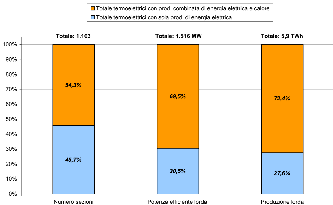
Figura 20: Impianti termoelettrici nell'ambito della GD.
