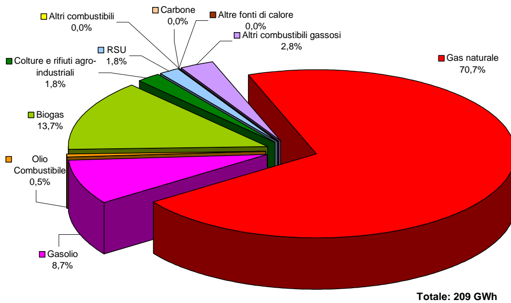
Figura 19 7 : Produzione di energia elettrica dalle diverse fonti utilizzate nell'ambito della MG da termoelettrico per la produzione combinata di energia elettrica e calore.
