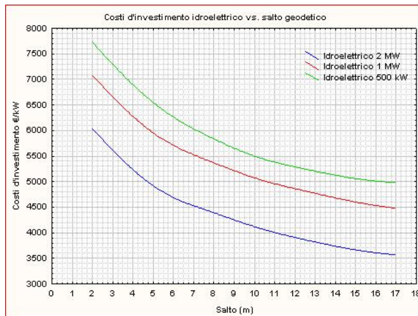
Figura 3.1: Costi di investimento tipici per gli impianti idroelettrici di piccola taglia.
