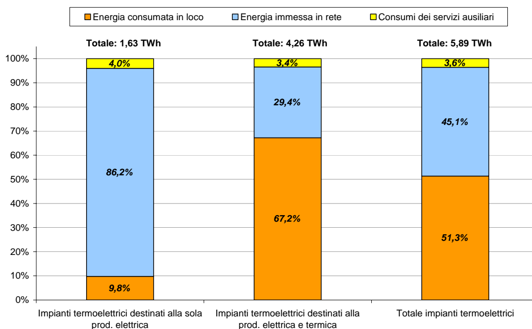
Figura 4.24: Ripartizione della produzione da impianti termoelettrici tra energia immessa in rete ed energia autoconsumata nell'ambito della GD.
