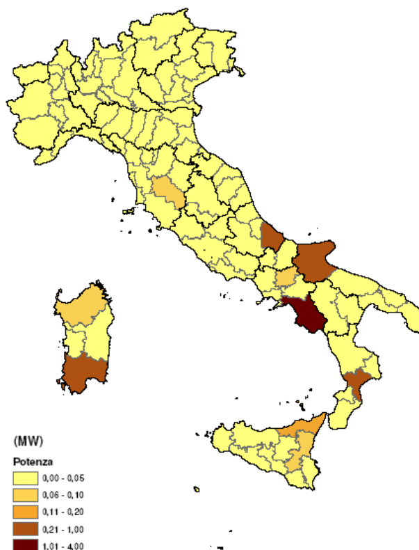
Figura 4.17: Dislocazione degli impianti fotovoltaici di GD in termini di potenza.
