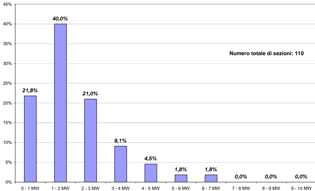
Figura 4.27: Distribuzione delle sezioni con turbine a vapore in contropressione per la produzione combinata di energia elettrica e calore tra le varie classi di potenza nell'ambito della GD.
