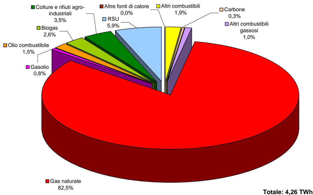
Figura 4.23 7 : Produzione di energia elettrica dalle diverse fonti utilizzate nell'ambito della generazione termoelettrica distribuita per la produzione combinata di energia elettrica e calore.
