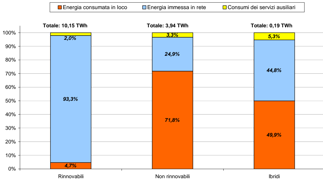
Figura 4.4: Ripartizione della produzione lorda da GD tra energia immessa in rete ed energia autoconsumata (per impianti alimentati da fonti rinnovabili, non rinnovabili e per impianti ibridi).
