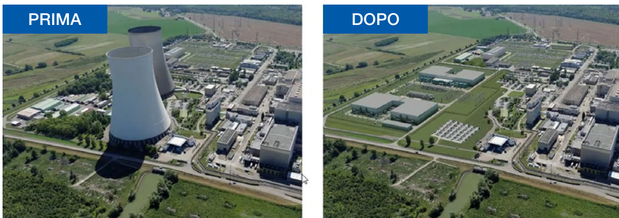
FIGURA 29 Sito esistente della centrale nucleare di Filisburgo dismessa per costruire le Stazioni di Conversione
